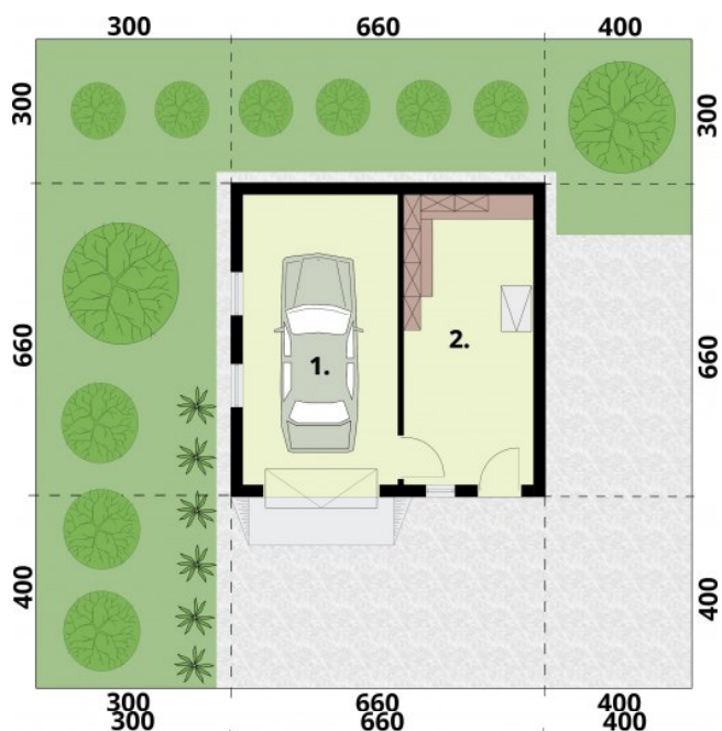
Rzut przyziemia
