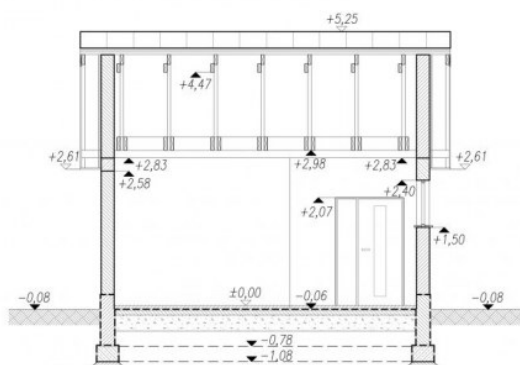
PRZEKRÓJ B-B
