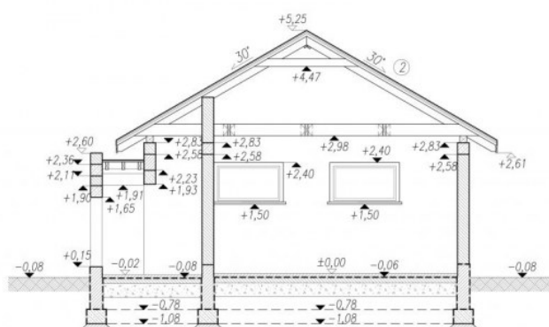
PRZEKRÓJ B-B
