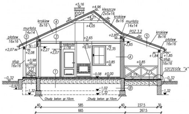
PRZEKRÓJ A-A
