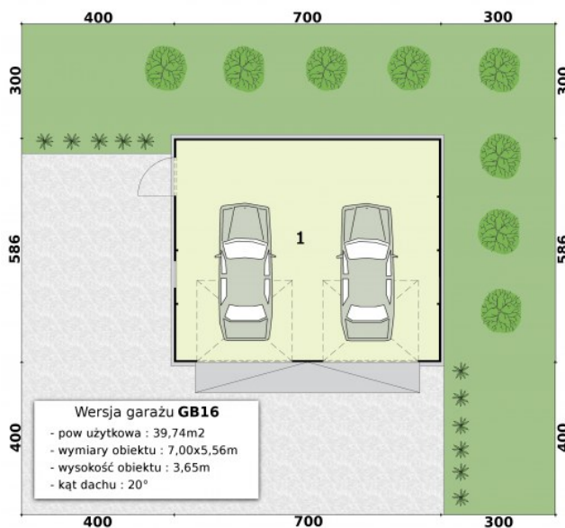
Rzut przyziemia garażu GB16
