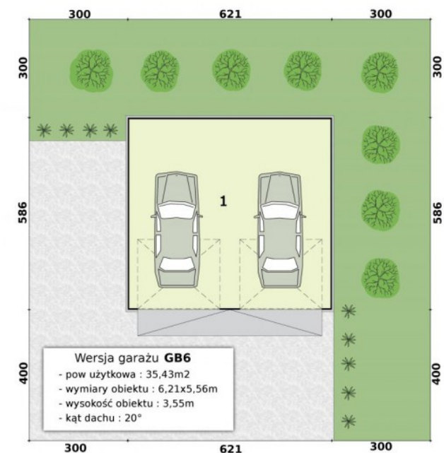
Rzut przyziemia garażu GB6
