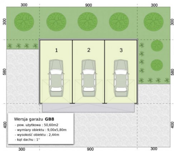
Rzut przyziemia garażu GB8
