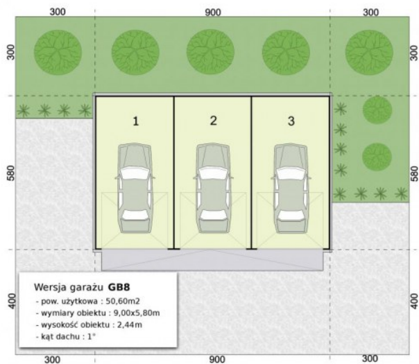
Rzut przyziemia garażu GB8
