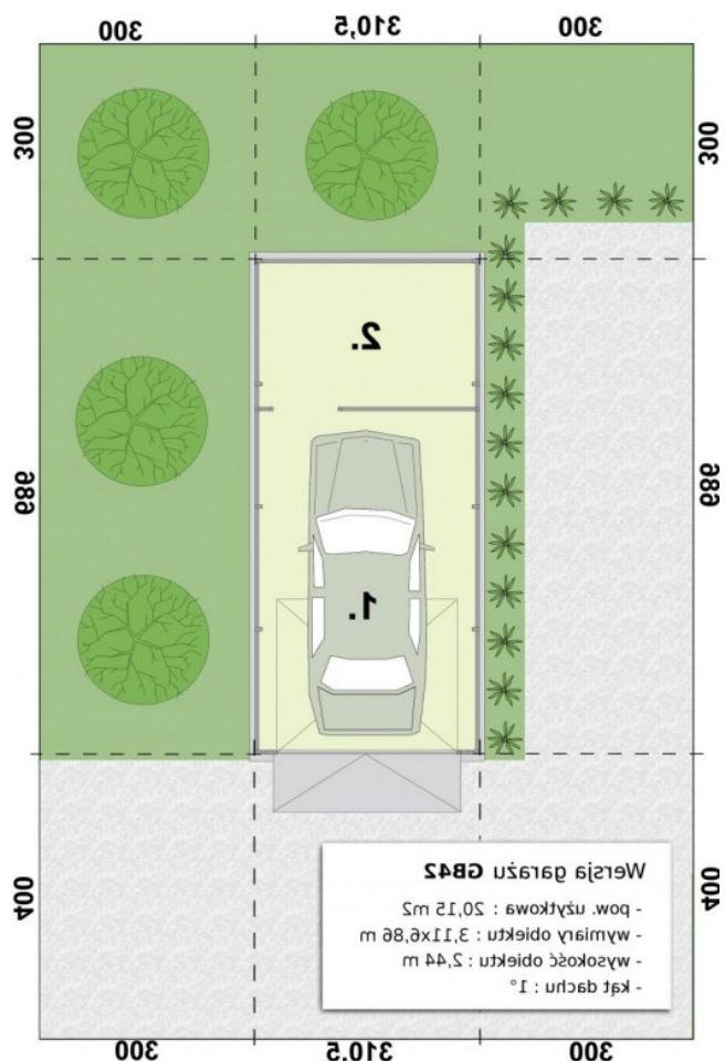
Rzut przyziemia
