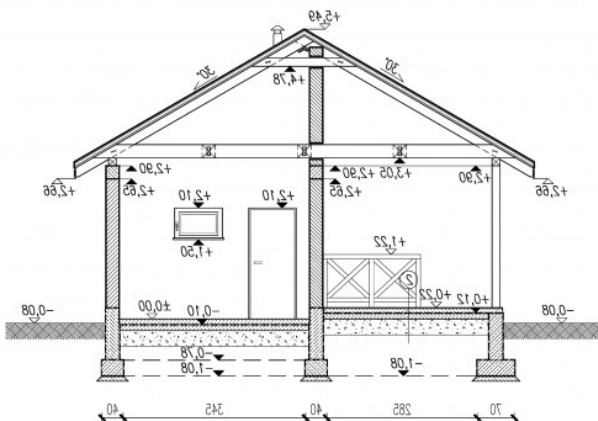
PRZEKROJ B-B
