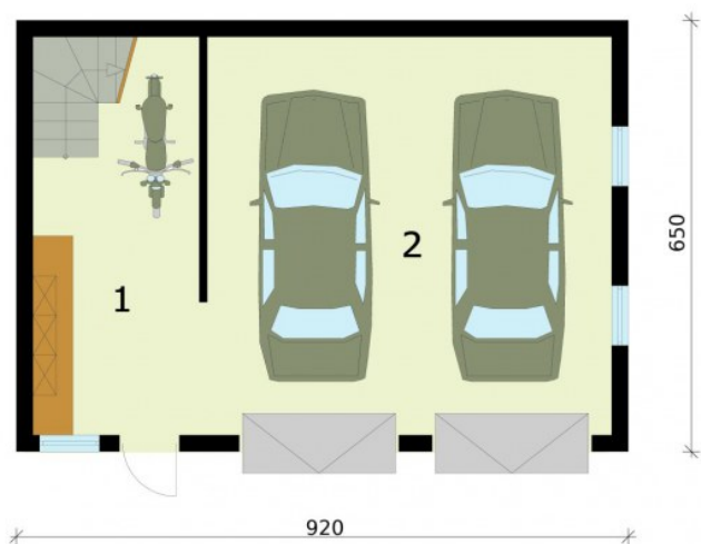
Rzut przyziemia
